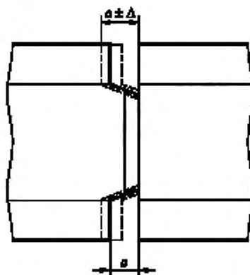
a — ширина зазора по клеевому соединению ящика
